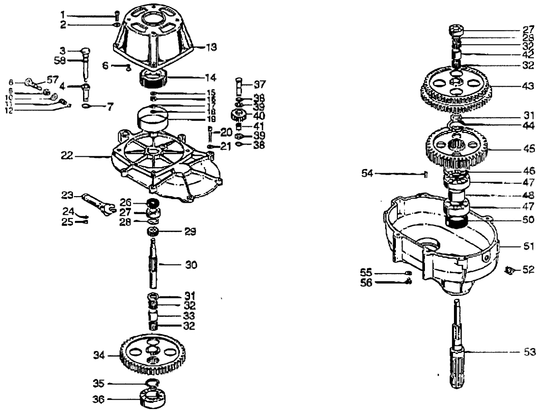
Gear box - Groupe réducteur - Gruppo riduttore
