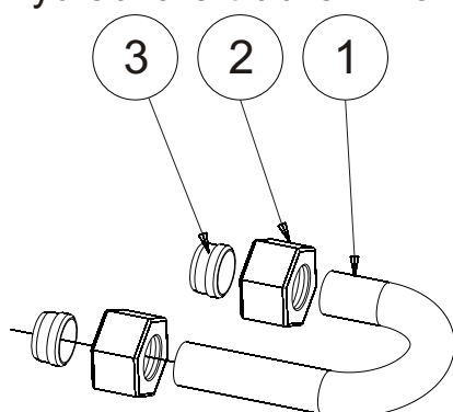
1S02K230 (No. 9) Hydraulická trubka A-komplet
