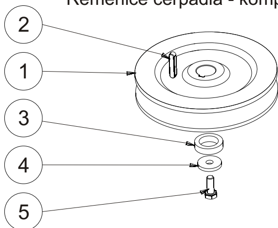
1S02K030 1S02K031 (No. 2) Řemenice čerpadla - komplet
