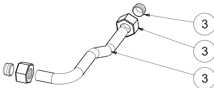
1S02K240 (No. 10) Hydraulická trubka B-komplet
